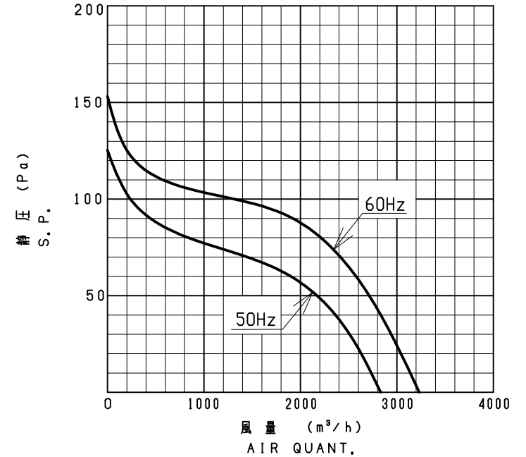
性能曲線 CHARACTERISTICS CURVE JIS C 9603 (+20°C)
