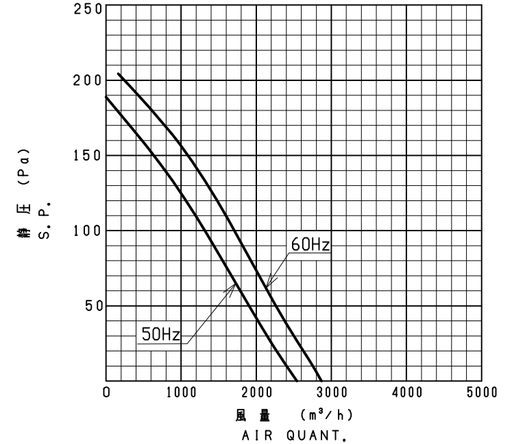
性能曲線 CHARACTERISTICS CURVE JIS C 9603 (+20℃)
