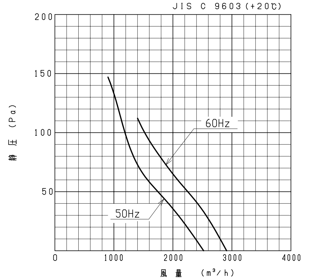
性能曲線
