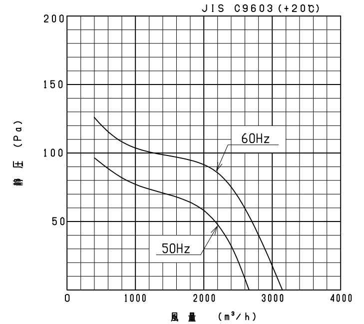
性能曲線 (Performance curve)
