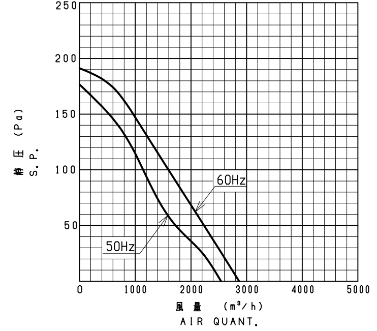
性能曲線 CHARACTERISTICS CURVE JIS C 9603 (+20℃)
