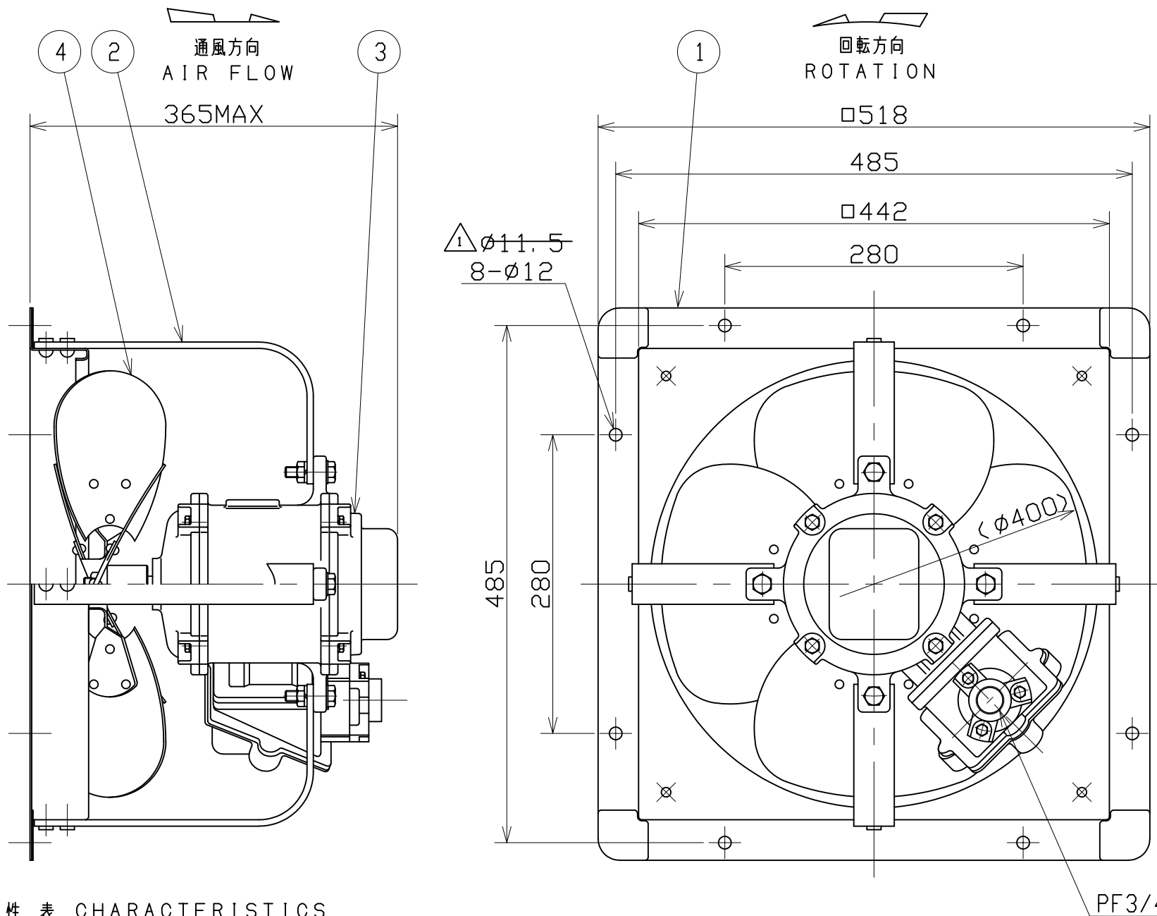
特性表 CHARACTERISTICS
