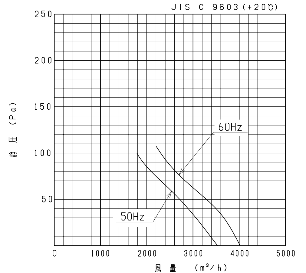
性能曲線
