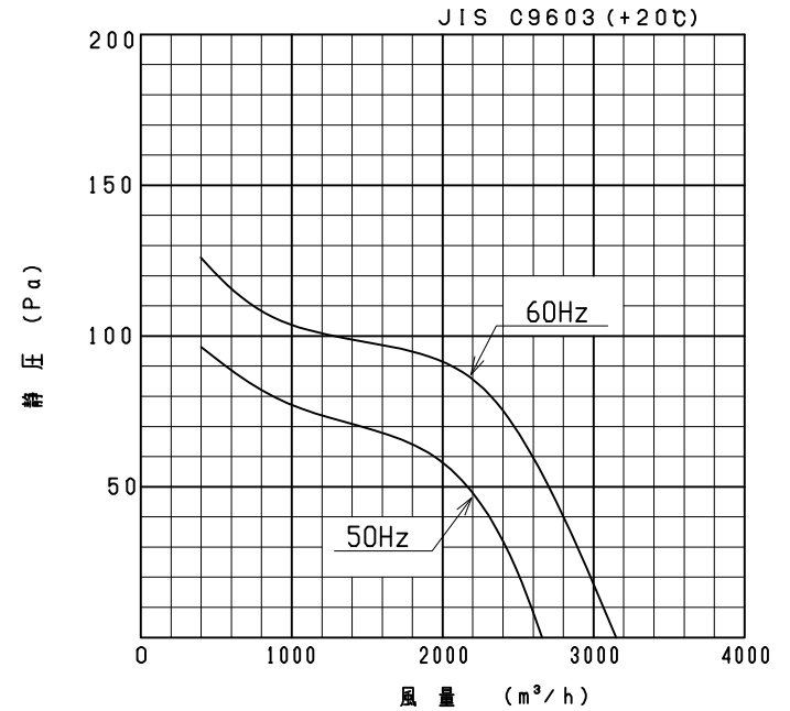
性能曲線
