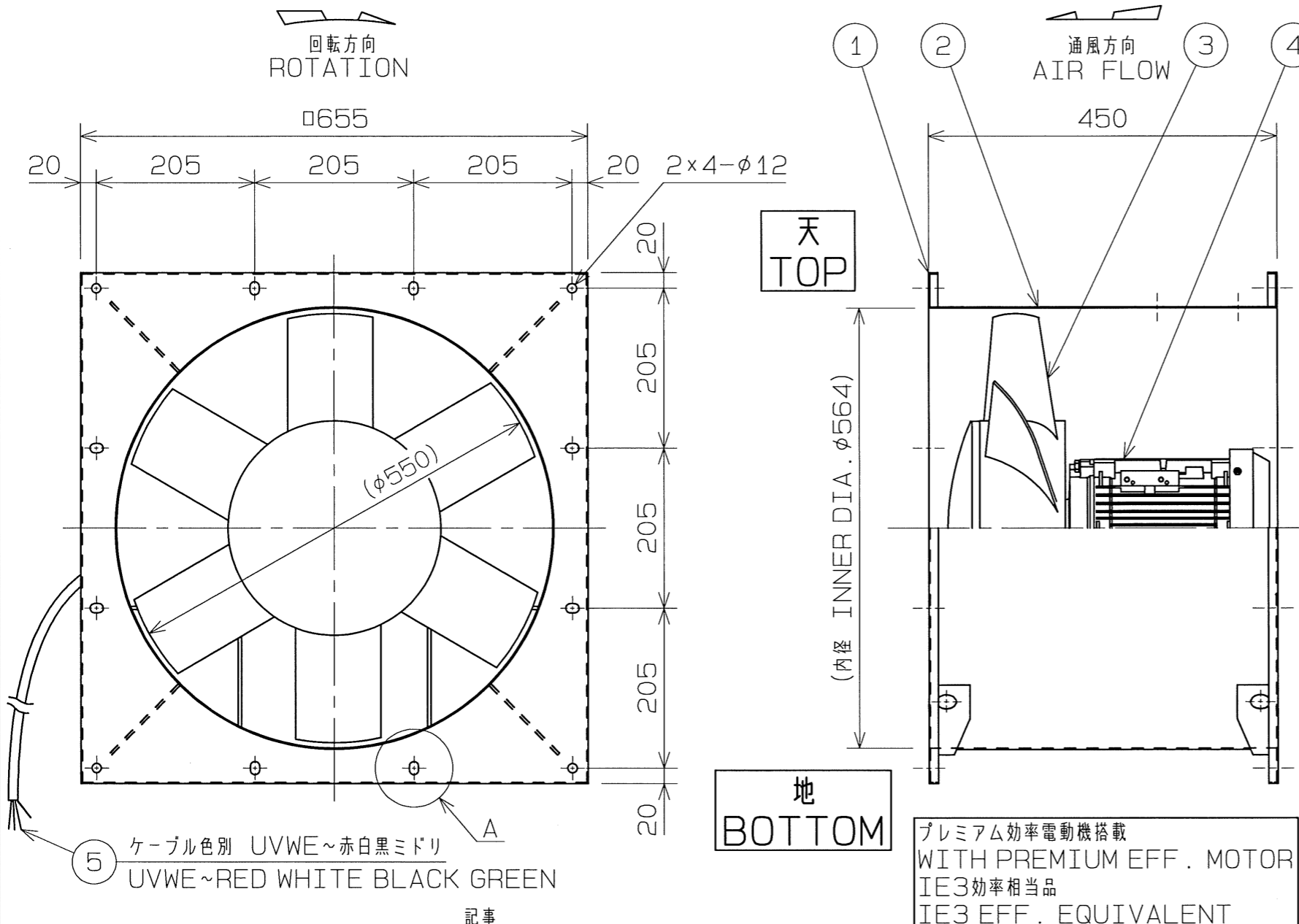
A部 詳細 DETAIL A
