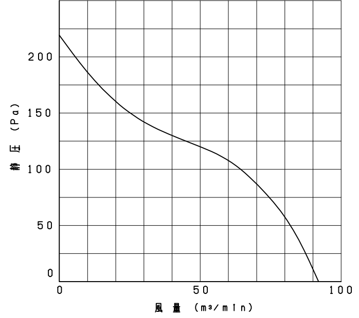
特性曲線 JIS B8330 (at 20℃)
